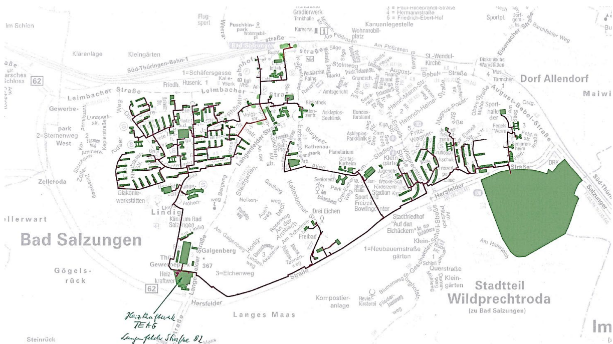
Abbildung 25: Übersicht über das Fernwärmenetz der TEAG in Bad Salzungen
